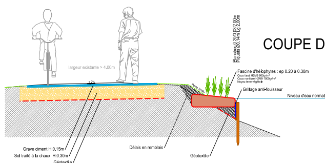
▲ Plan de coupe du projet de tronçon Dieue-Haudainville
